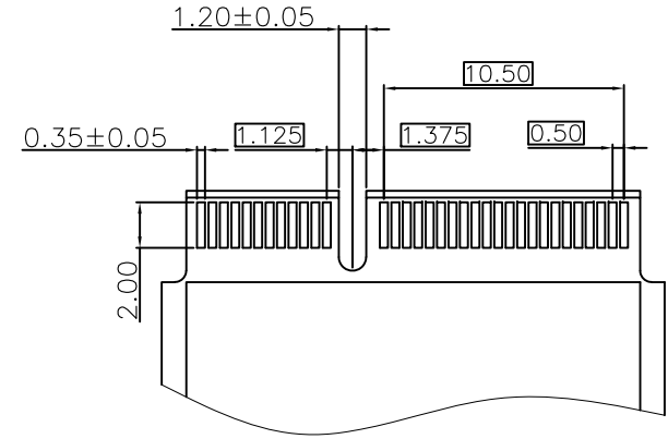
TOP SIDE
